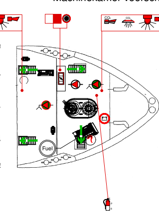
Machiniekamer voorschip
