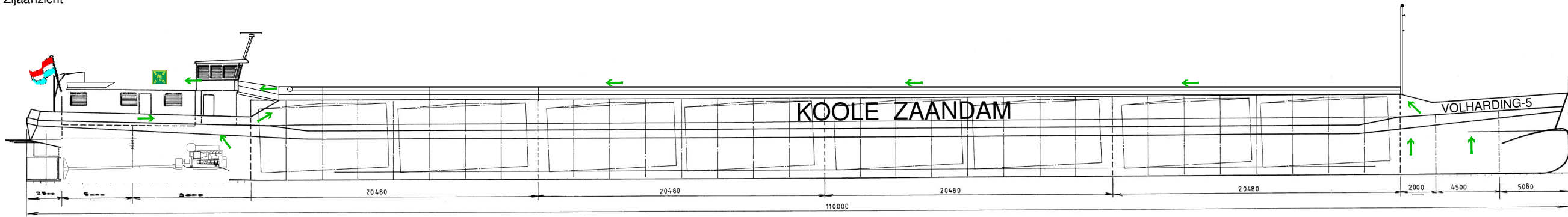
Zijaanzicht
